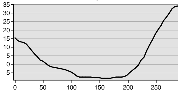
Stornorrfors, sektion 24
