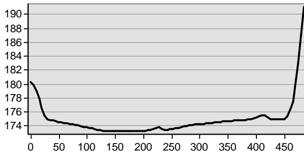
Tuggen, sektion 16
